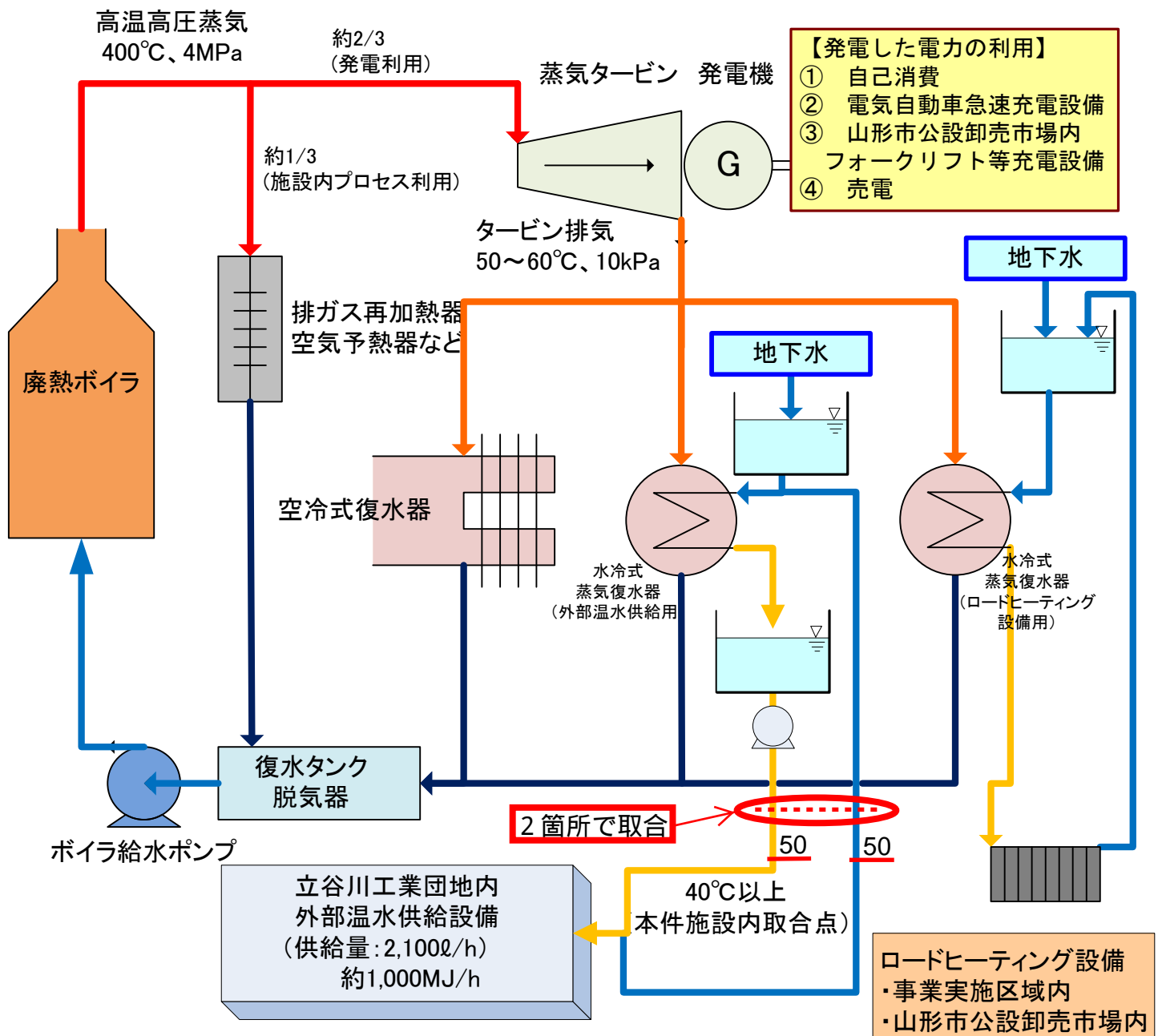
図 エネルギー回収施設(立谷川)における余熱利用のイメージ
